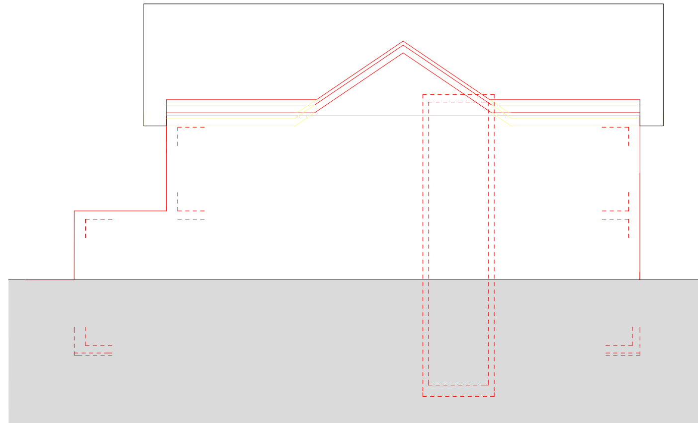
PROSPETTO EST
